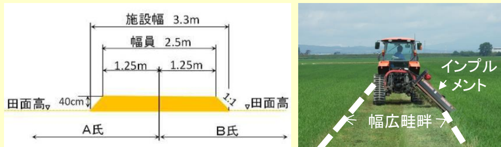
図-4.3.11 幅広畦畔の事例
