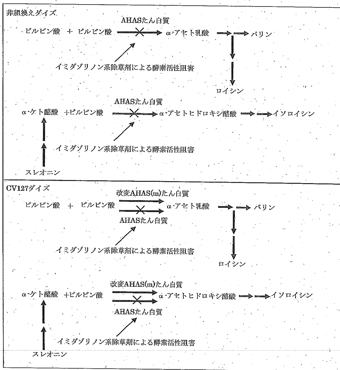
図 改変 AHAS(m)たん白質の作用機構
