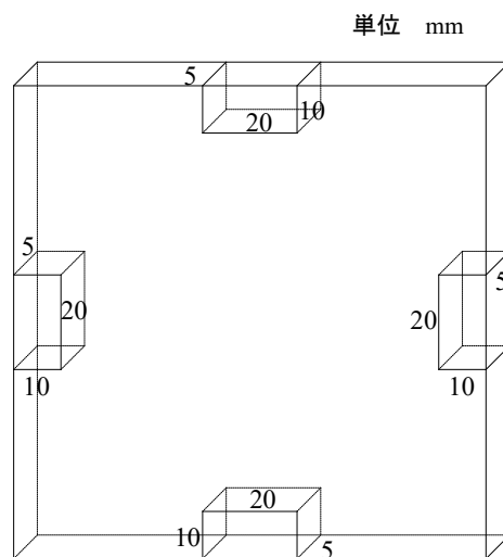
図 28－吸収量試験の木片採取位置
