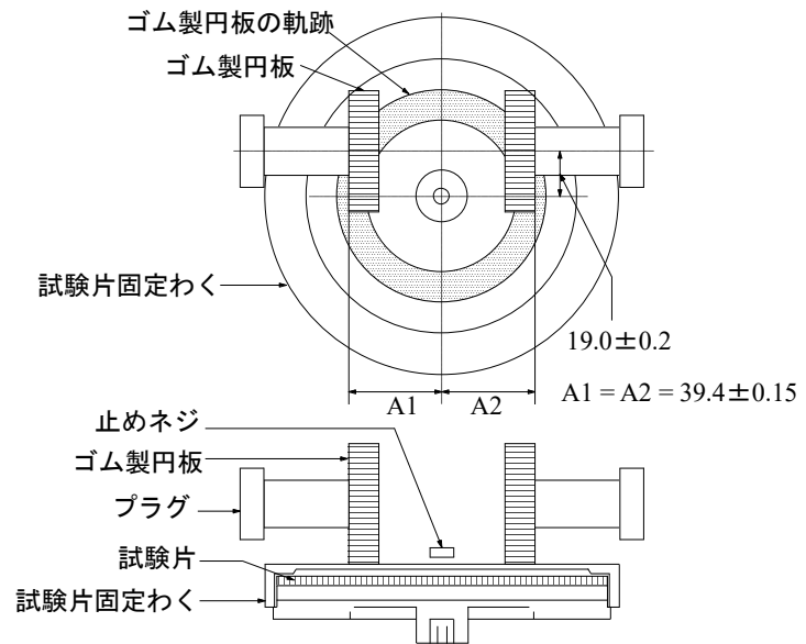
図 5-1 摩耗試験の方法 2
