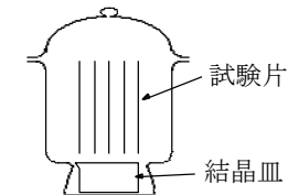
図3—ホルムアルデヒドの捕集方法
