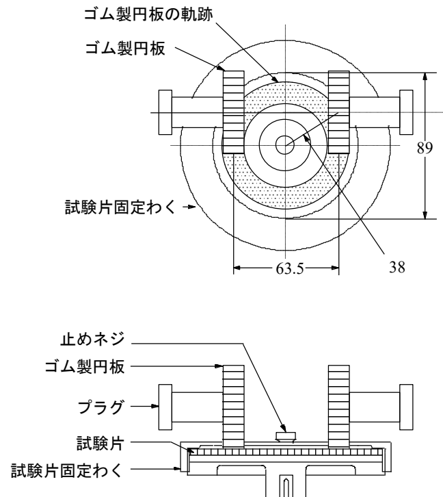
図 4－摩耗試験の方法 1
