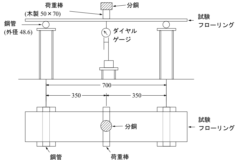
図3ー曲げ試験の方法
