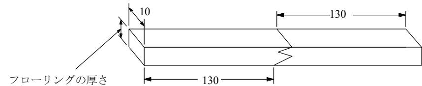
図1-曲げ強度試験の試験片
