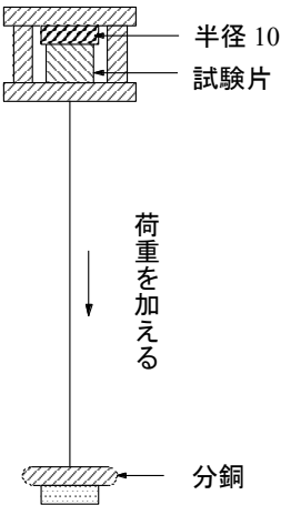
b) 側面図
