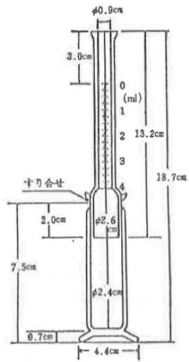
図 2—ガス定量器
