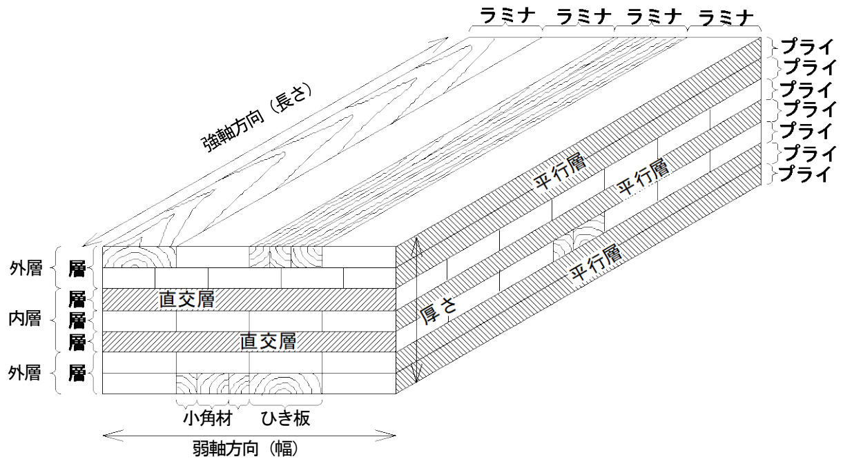
図1—各部の名称 (5層7プライのもの。)
