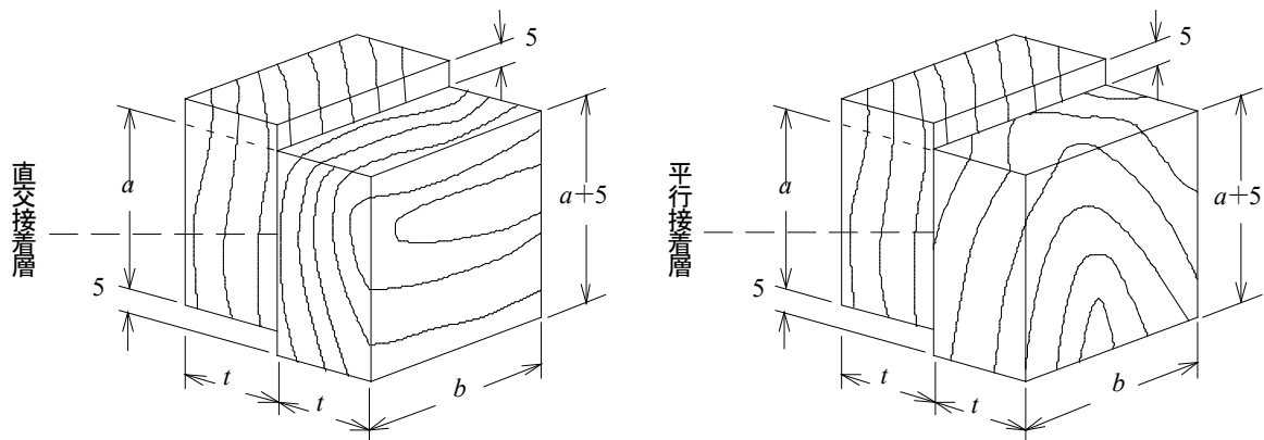
図 11—ブロックせん断試験用試験片 (直交接着層及び平行接着層用)
