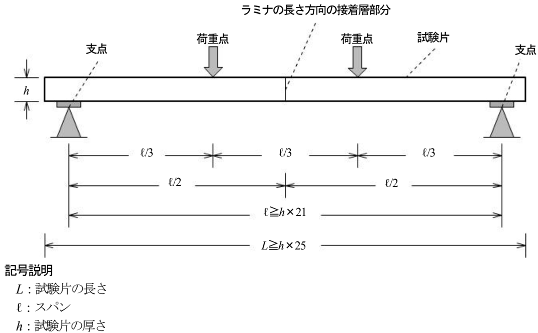
図 17—ラミナの曲げ C 試験の方法
