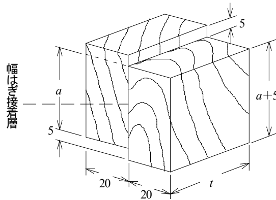
図 12—ブロックせん断試験用試験片 (幅はぎ接着層用)
