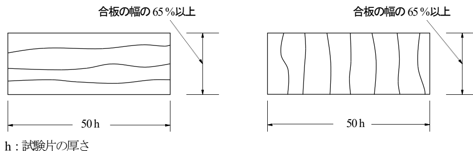
図8—試験片の作製方法（ラワン以外用）
