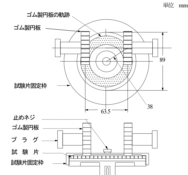
図 14－摩耗試験の方法 1
