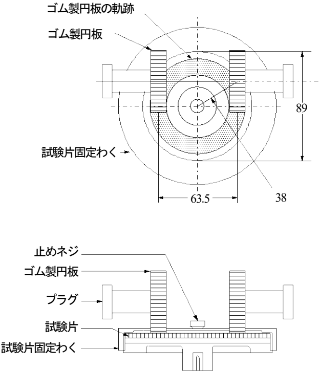
図 4—摩耗試験の方法 1
