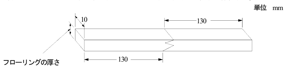
図1—曲げ強度試験の試験片
