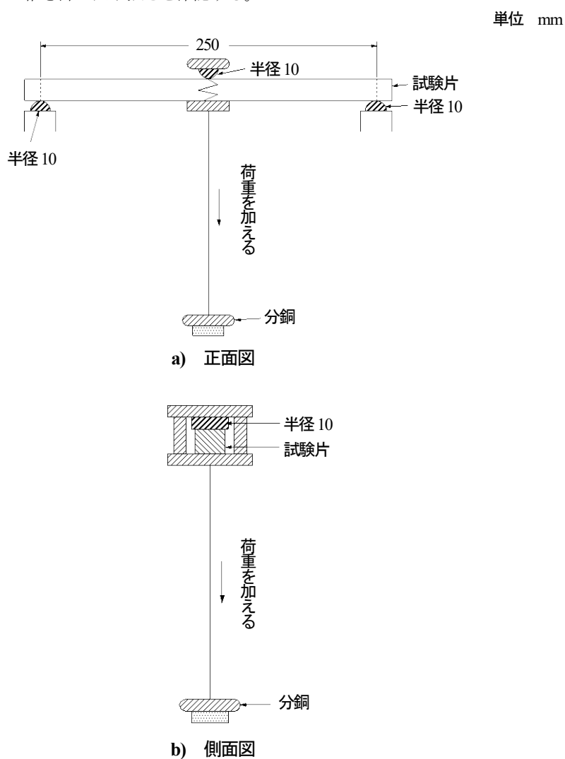
図2—曲げ強度試験の方法
