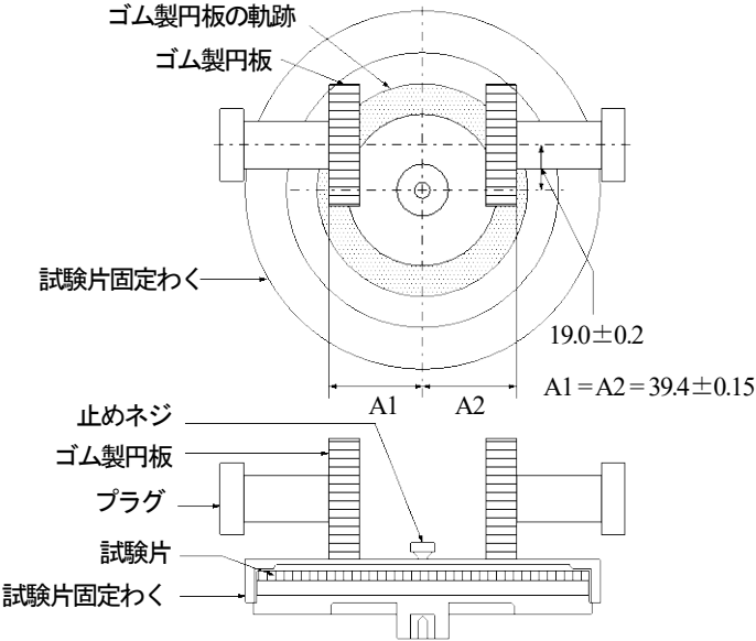
図 5—摩耗試験の方法 2
