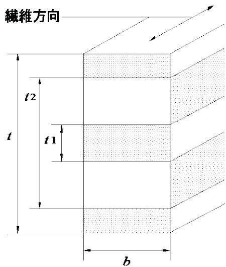
図 1—有効断面係数比（5 層の場合）
