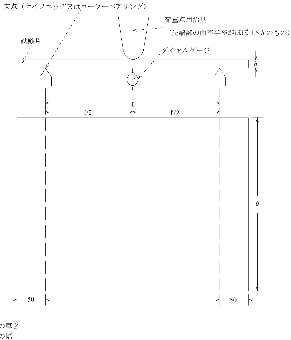
図3—曲げ試験の方法
