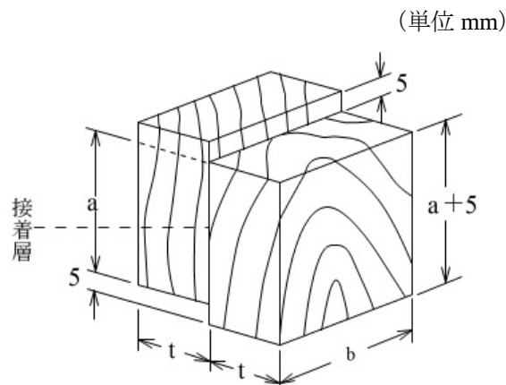
図17ーブロックせん断試験用試験片(いす型)
