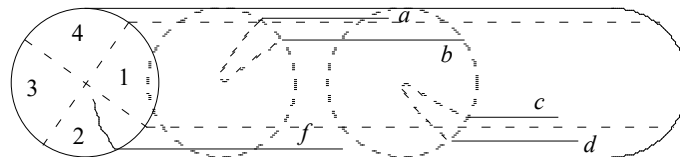
図 29—隣接材面の貫通割れ
