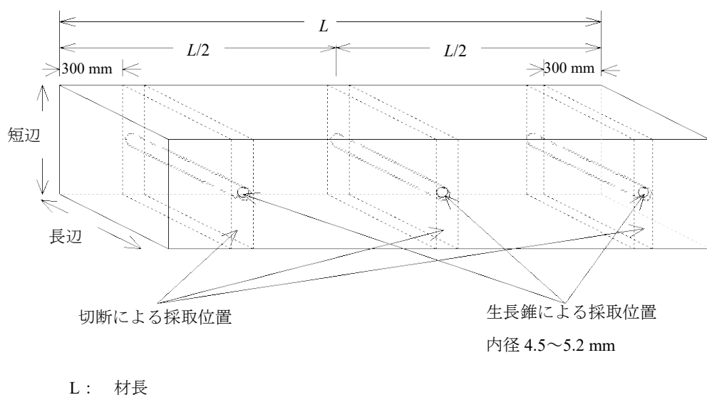
図 42—含水率試験片採取位置（例）
