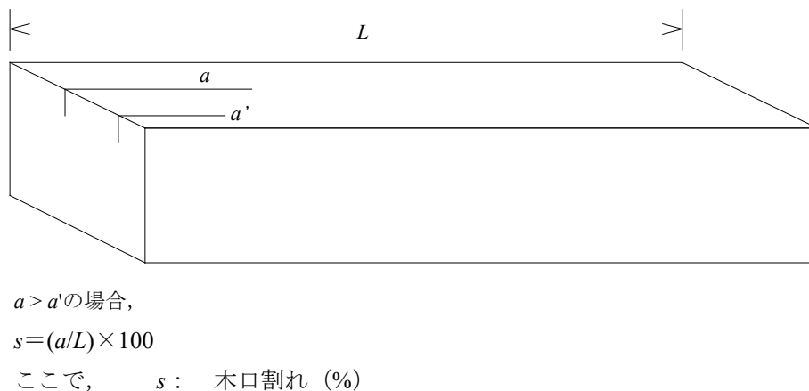
図 32—同一木口に 2 個以上ある場合
