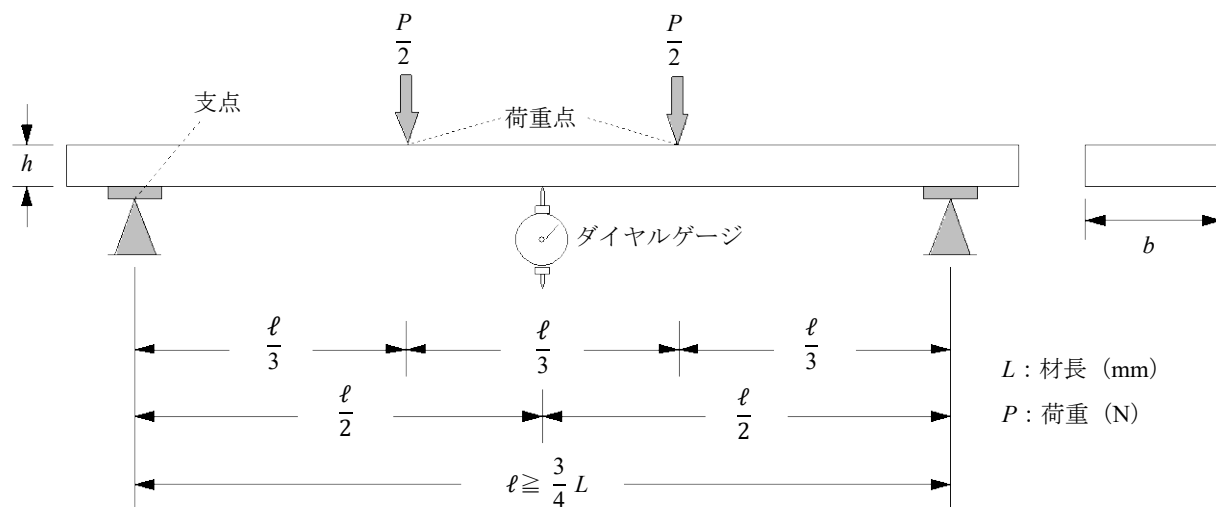
図 43—曲げ試験
