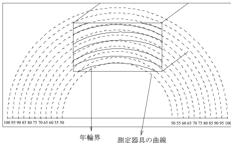
図 41—髓心部の測定方法
