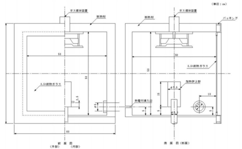
図 8 かくはん箱
