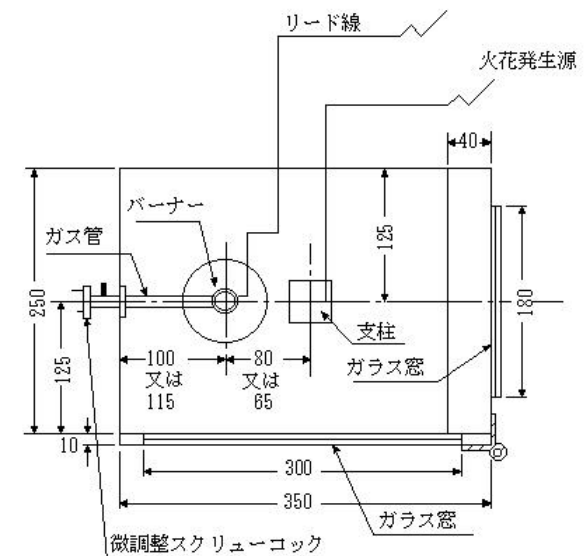
図1.4 電気火花発生装置
