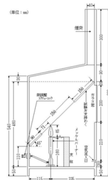
図 1 2 燃焼試験箱
