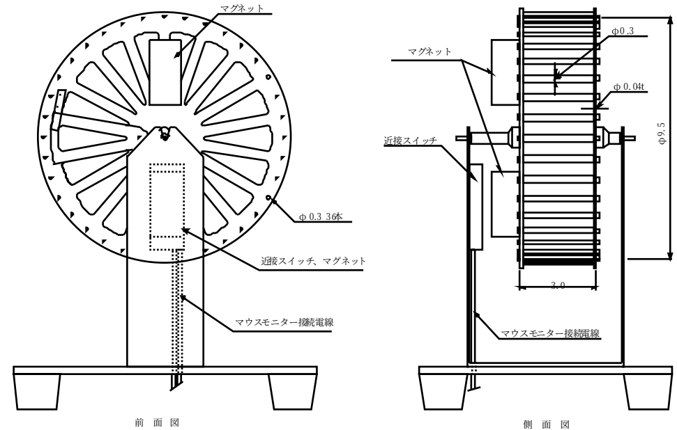
図10 回転かご
