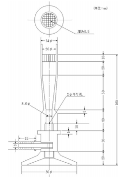
図15 ムッケルバーナー
