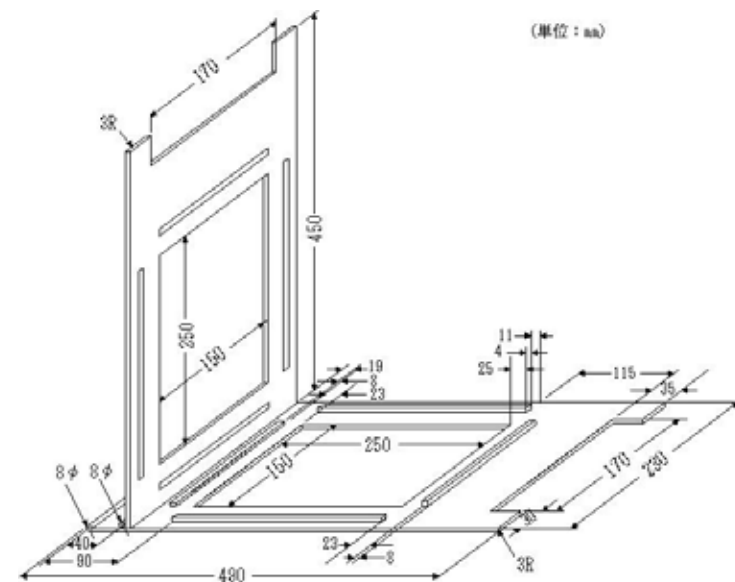
図1.4 電気火花発生装置
