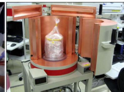
ゲルマニウム半導体 検出器による放射性物 質分析
