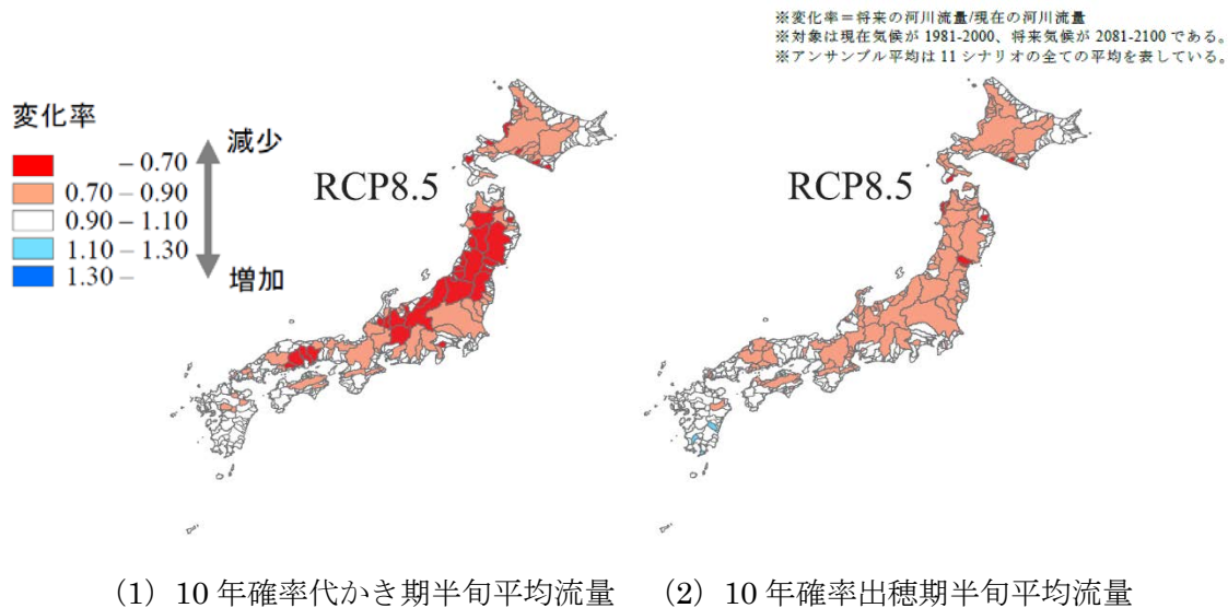
図 3.5-73 農業水利用に対する全国影響評価マップ
