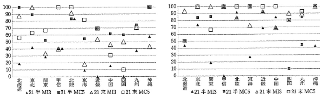
図 3.5-77 被災率による将来リスクが高まる地域割合 (%) (左：50年降雨 RCP2.6, 右：50年降雨 RCP8.5) 253
