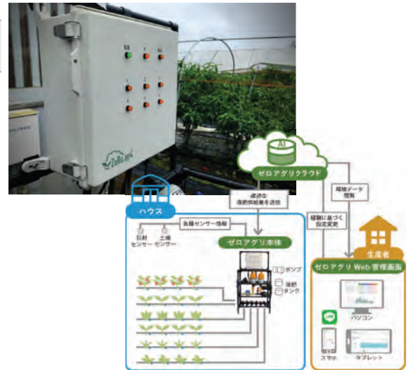
自動灌水施肥装置
