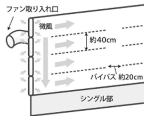
W快適エアカーテンの基本構成
