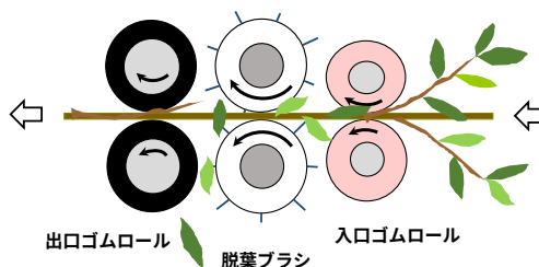
脱葉部の構成(真横から)
