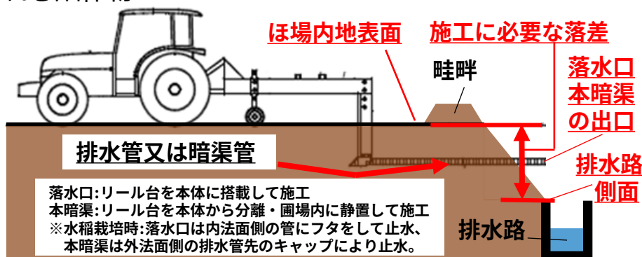
排水管理設置の仕組み（特許第6899113号）
