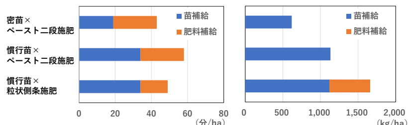
図 施肥田植時の作業性比較（苗と肥料の補給時間、苗と肥料の運搬重量）
