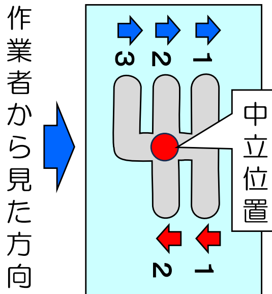
停車時の変速レバーの位置
