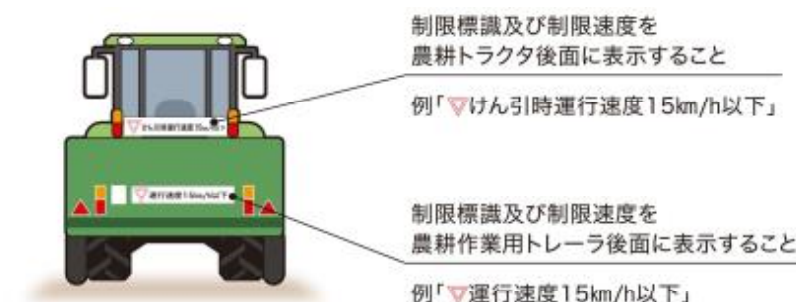
図2-4-7 傾斜角一定以下、ブレーキ未装備トレーラーに必要な表示
