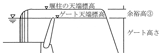
堰柱天端標高説明図
