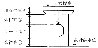
堰柱天端標高説明図
