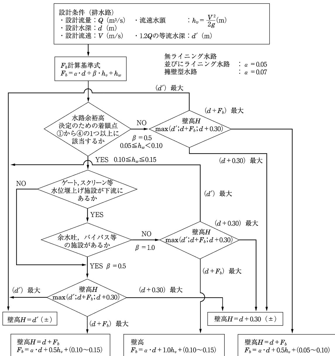
図-6.6.3 排水路（開水路）水路余裕高算定と水路壁高決定のフローチャート
