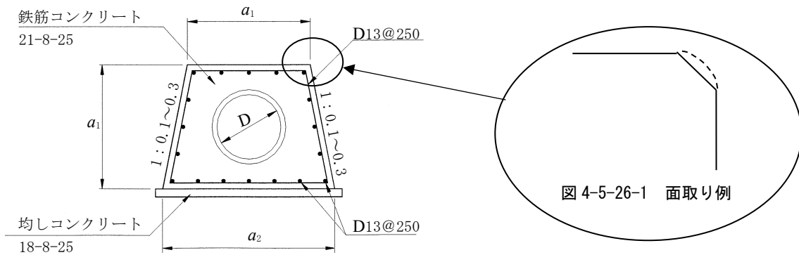
図4-5-26 底樋の設計例
