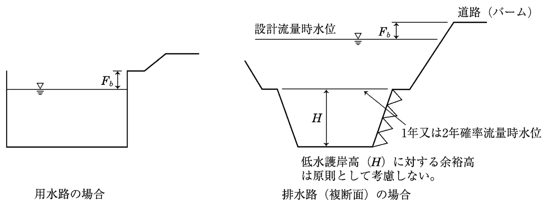
図-6.6.1 水路の余裕高
