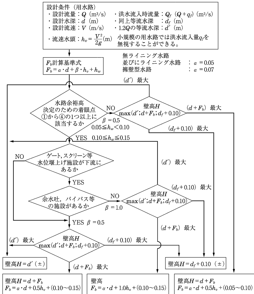
図-6.6.2 用水路（開水路）水路余裕高算定と水路壁高決定のフローチャート
