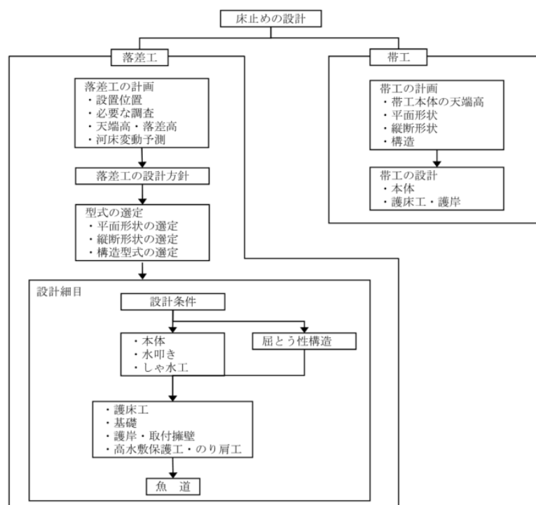
図 10-1-2 床止めの設計手順
