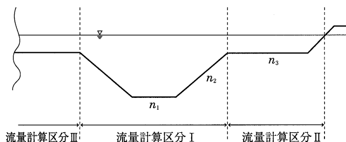
図-6.2.2 流量計算区分図
