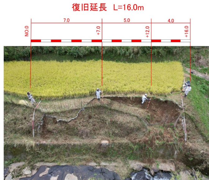
写真 2-12-4 UAV（ドローン）による全景写真（農地災その 2）
