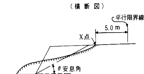
図 3-2-2 復旧すべき農地面積
