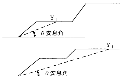
図 3-2-3 安息角が筆界を越えた場合の復旧すべき農地面積
