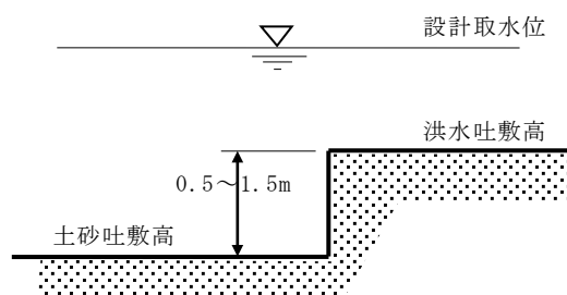
図 5-5-4 洪水吐の標準敷高
