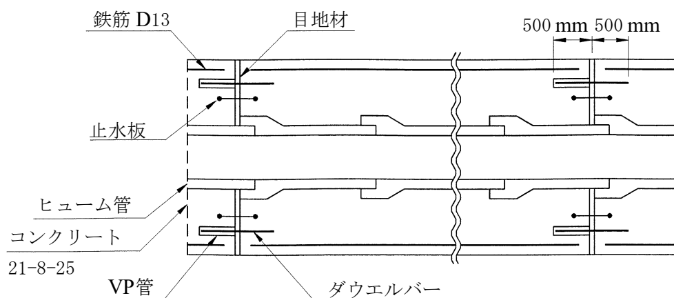
図 4-5-28 底樋の継手構造例
