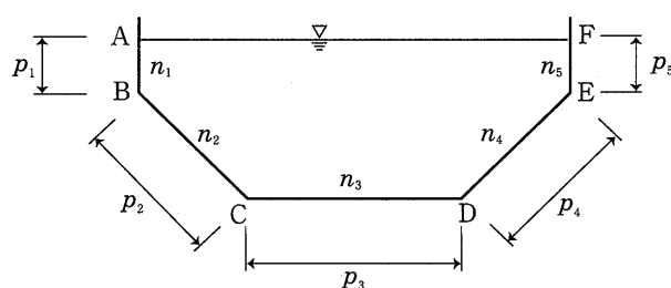
図 6-5-1 潤辺図
