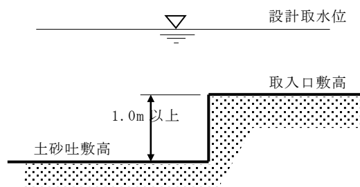
図 5-5-3 土砂吐の標準敷高
