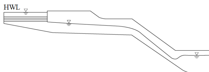
図 4-5-12 洪水吐の型式
