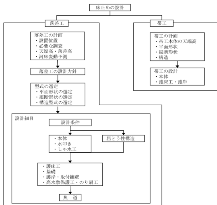
図 6-5-7 床止めの設計手順
