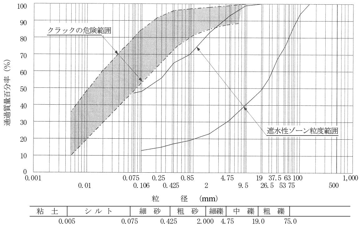
図 4-5-3 フィル材料の粒度範囲
