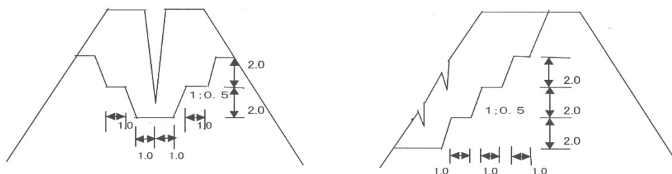
図 4-5-1 き裂の掘削例
