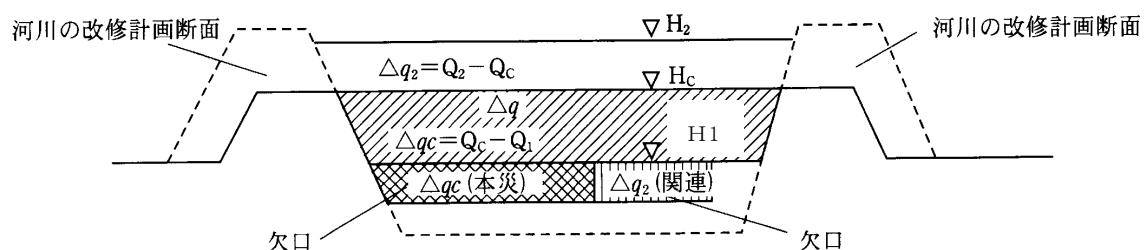
図 5-4-2 復旧対象洪水量 ( Q_2 ) が越水する場合
