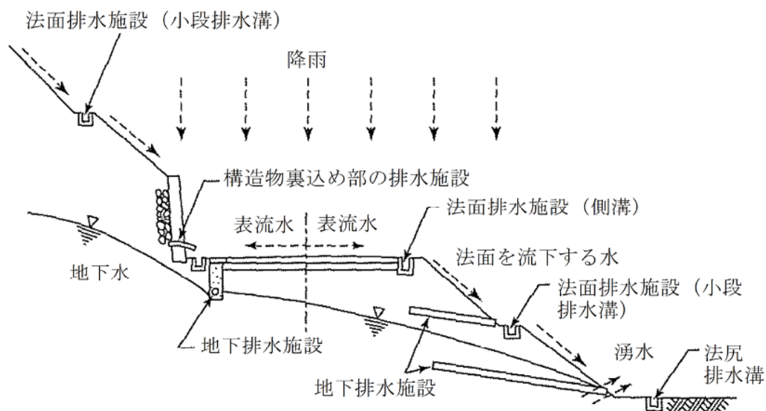
図 7-5-6 排水の構成
