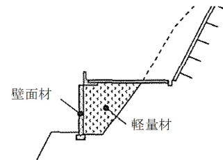
⑨軽量材を用いた擁壁
