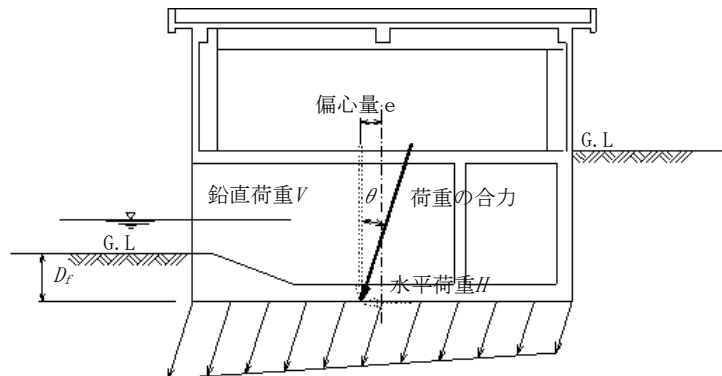
図 11-3-3 傾斜・偏心荷重
