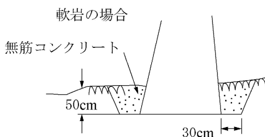
図 11-4-16 根入れ及び岩切付
