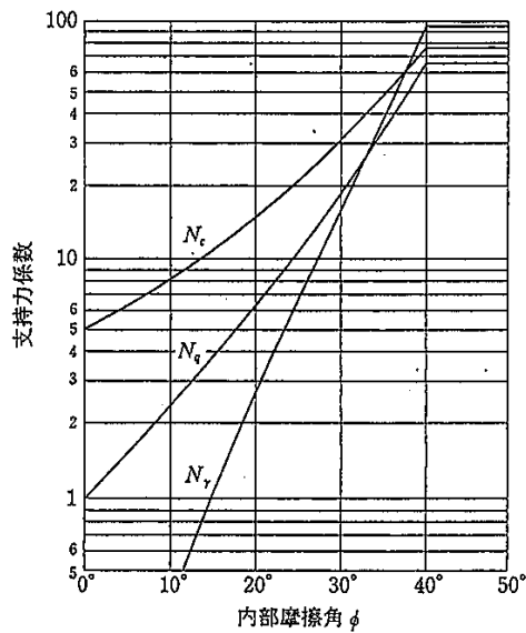
図 11-3-2 設計用支持力係数
