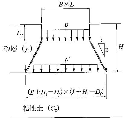
図 11-3-6 砂層の下に粘性土がある場合の略算法
