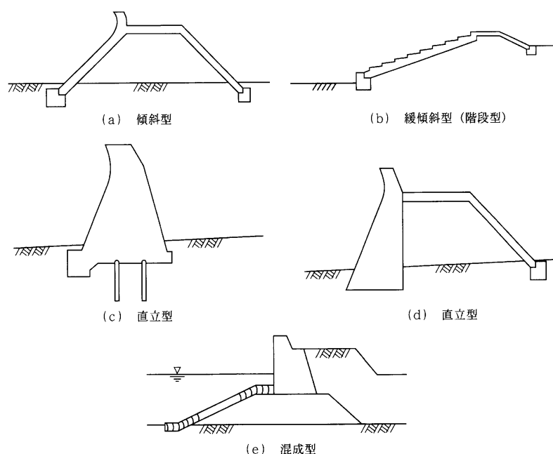
図 10-4-3 堤防の型式
