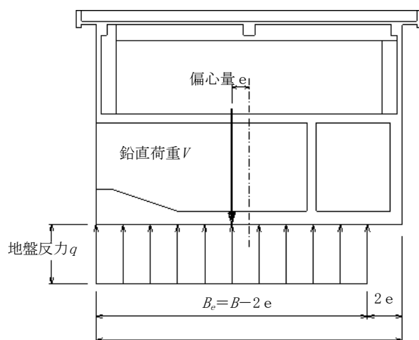
図 11-3-4 偏心荷重の有効載荷幅
