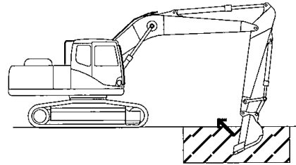
(a) 原位置混合処理方式の施工方法
