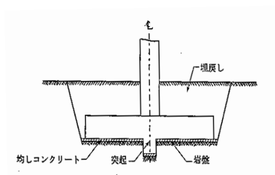
図 11-3-9 岩盤の場合（突起をつける場合）
