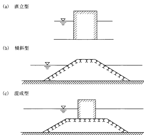
図 10-4-9 突堤の型式
