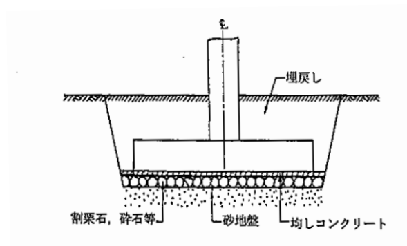
図 11-3-8 砂地盤の場合
