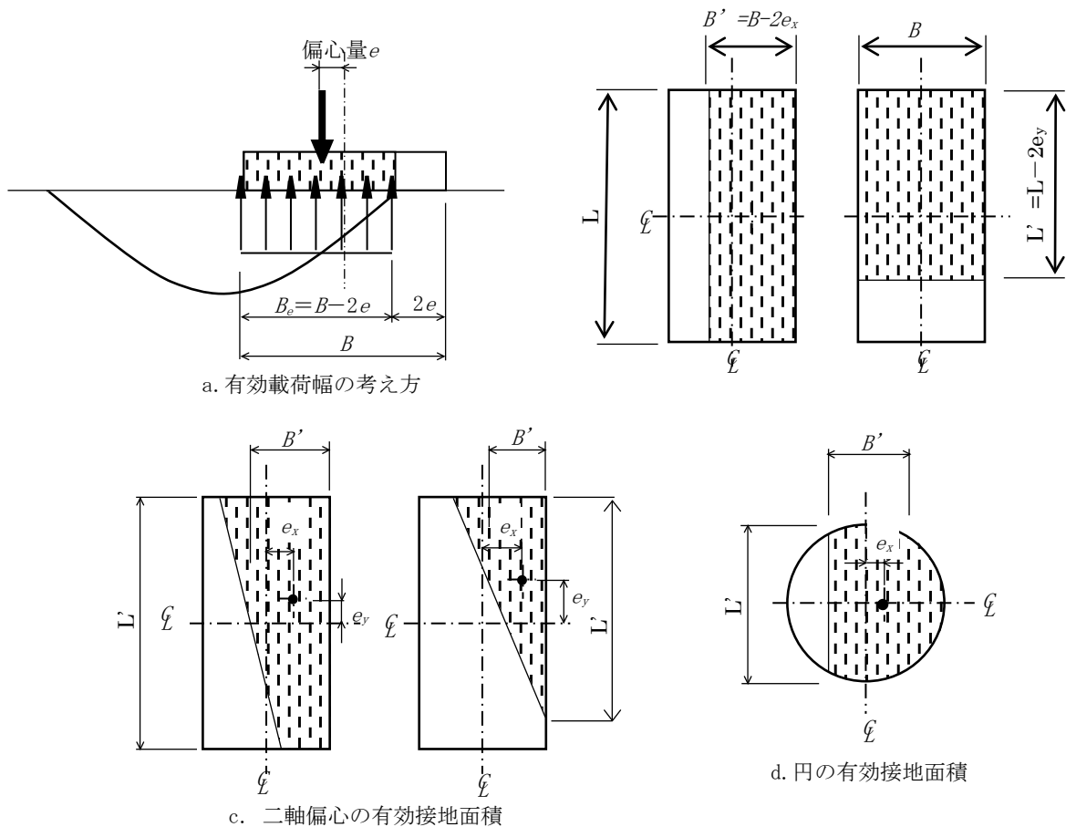
図 11-3-5 荷重に偏心のある場合の有効幅 ( B_e )、有効載荷幅 ( A_e )
