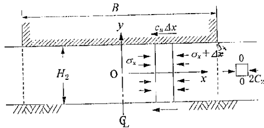
図 11-3-7 層厚が薄い軟弱粘性土層をはさむ場合の絞り出し破壊
