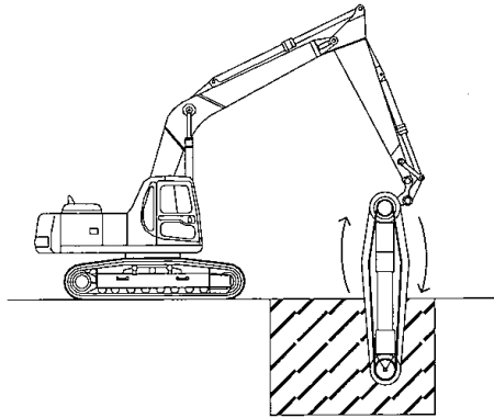
(a) 原位置混合処理方式の施工方法
