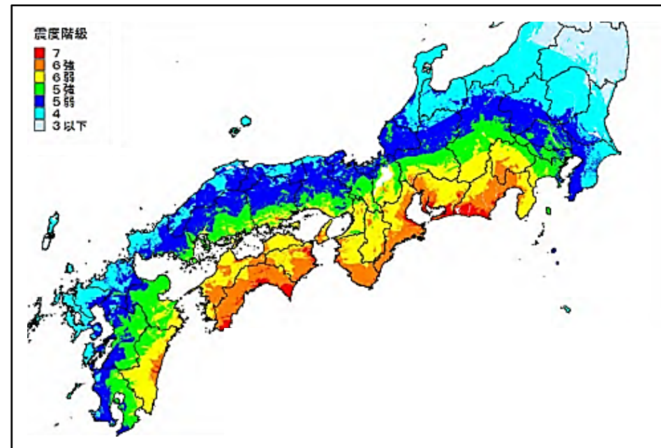
出典：内閣府「南海トラフの巨大地震による津波高・浸水域等（第二次報告）及び被害想定（第一次報告）について」資料1-1
