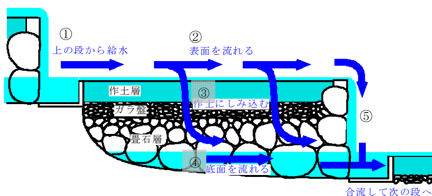
図 14 畳石式わさび田の構造と水の動き
