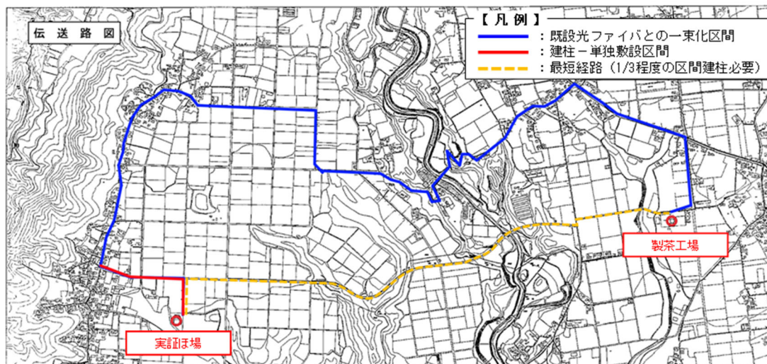
光ファイバの敷設計画
