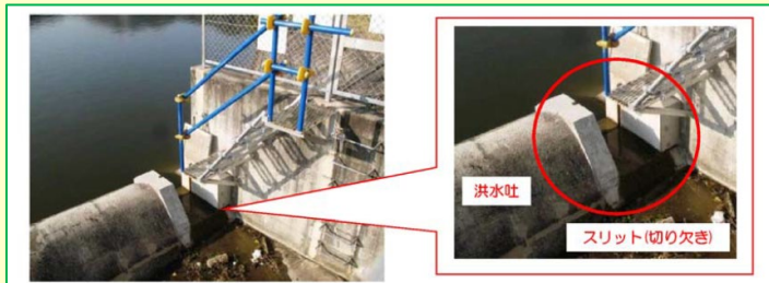
農業用ため池の洪水調節機能を強化するための「洪水吐きスリット」設置状況
