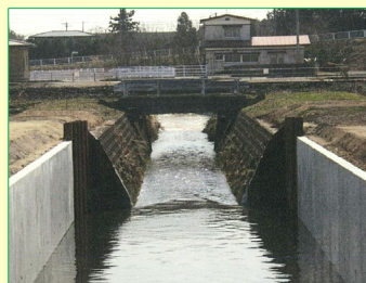
排水路の整備前 (排水能力 Q=16.3\text{m}^3/\text{s} )
