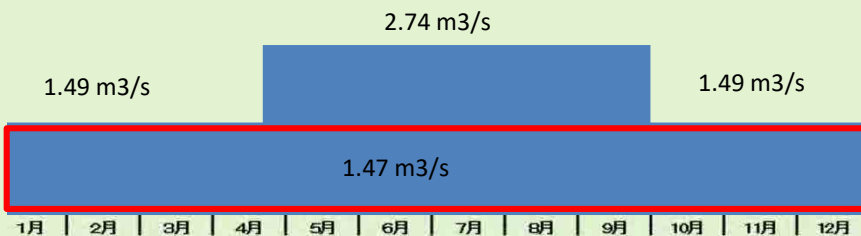
発電用水(農業用水に従属) ※最大発電使用量
