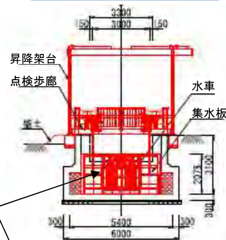
発電施設断面図
