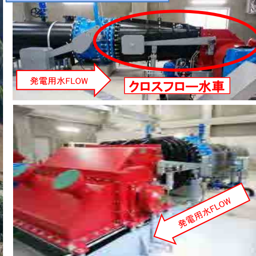
発 電 用 水 車
