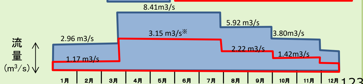
発電用水(農業用水に從属) ※最大発電使用量
