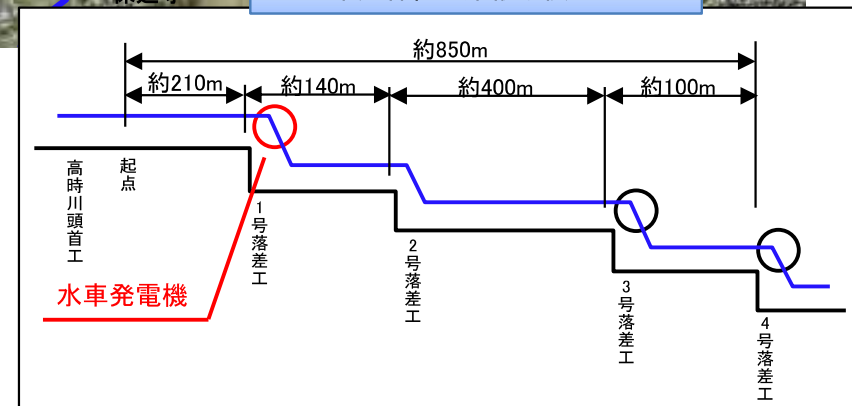
中央幹線水路縦断模式図
