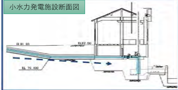
小水力発電施設
