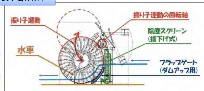
振り子式下掛け水車
