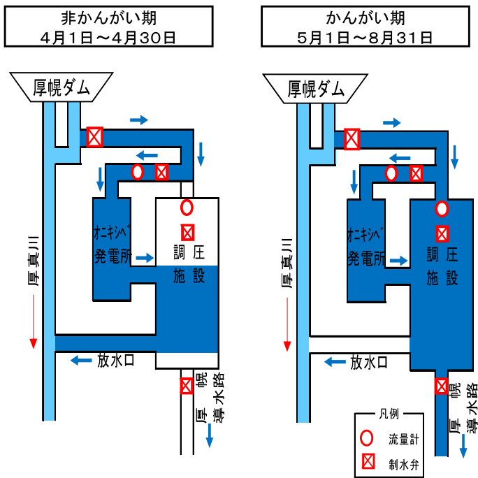
模 式 図
