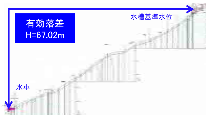
吉野小水力発電所 縦断面図
