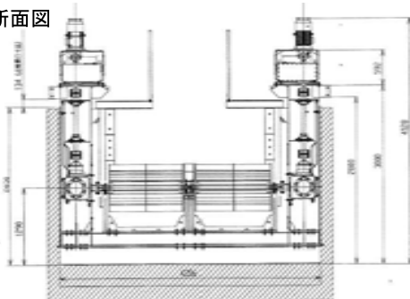
横断面図
