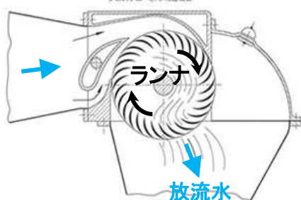
クロスフロー水車 構 造 概 要
