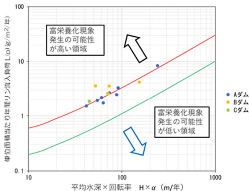
図2 ケーススタディダムの Vollenweider モデル計算結果
