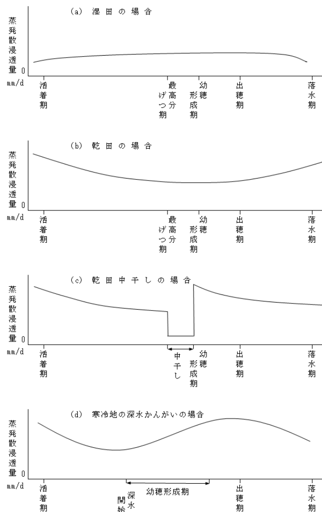
図-7.1 蒸発散浸透量（減水深）の標準的期別変化
