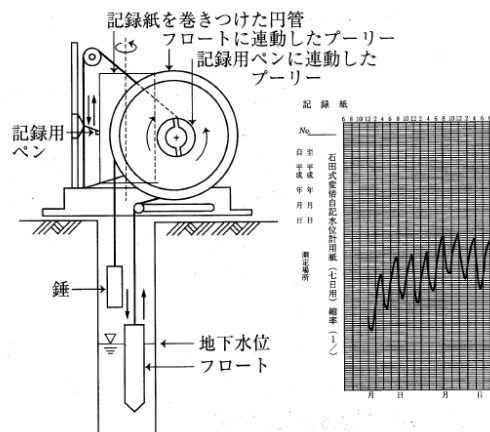
図-6.22 フロート式水位計（ペン書記録）による計測
