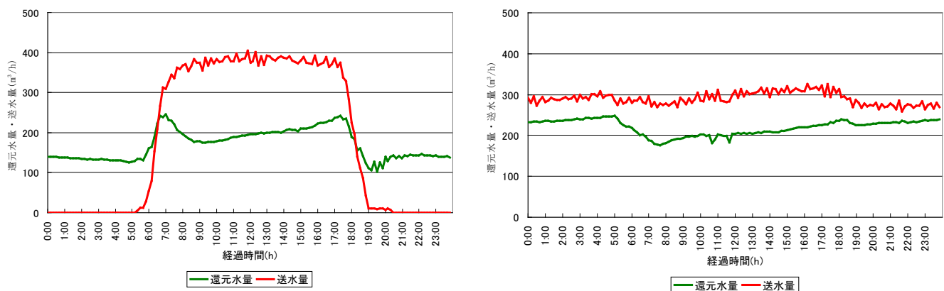
図-20.11 還元水量と送水量の時間変化
