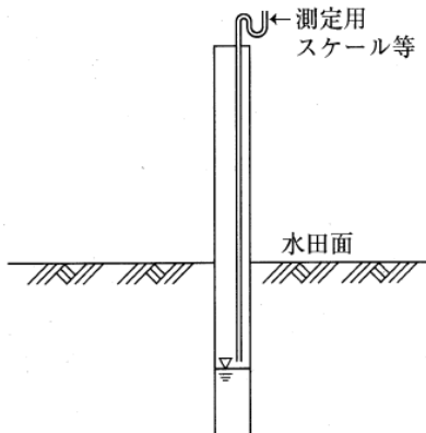
図-6.20 手測による測定
