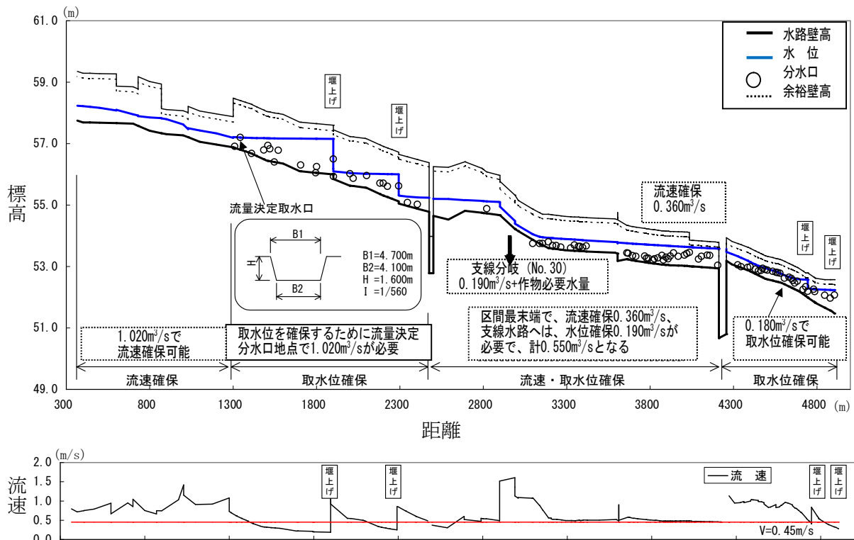
図-9.2 現況ケースでの検討結果（水位確保流量 1.020 \text{ m}^3/\text{s} ）
