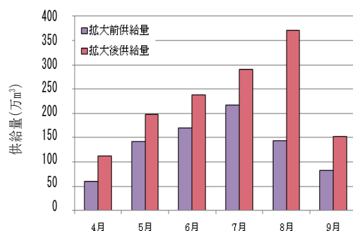
図-20.4 調整池拡大前と拡大後の供給量
