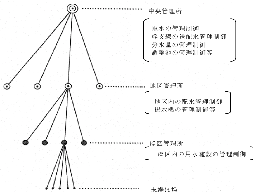
図-21.1 管理制御システムの分割と機能分担
