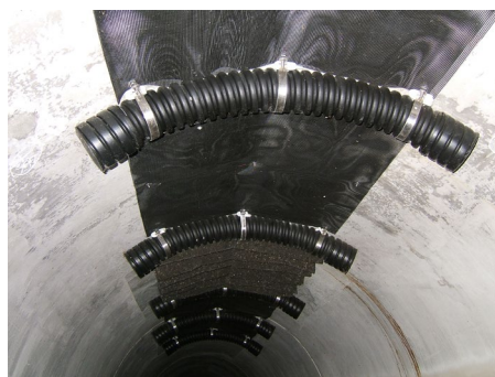
写真-14.9 設置後のコウモリピット
