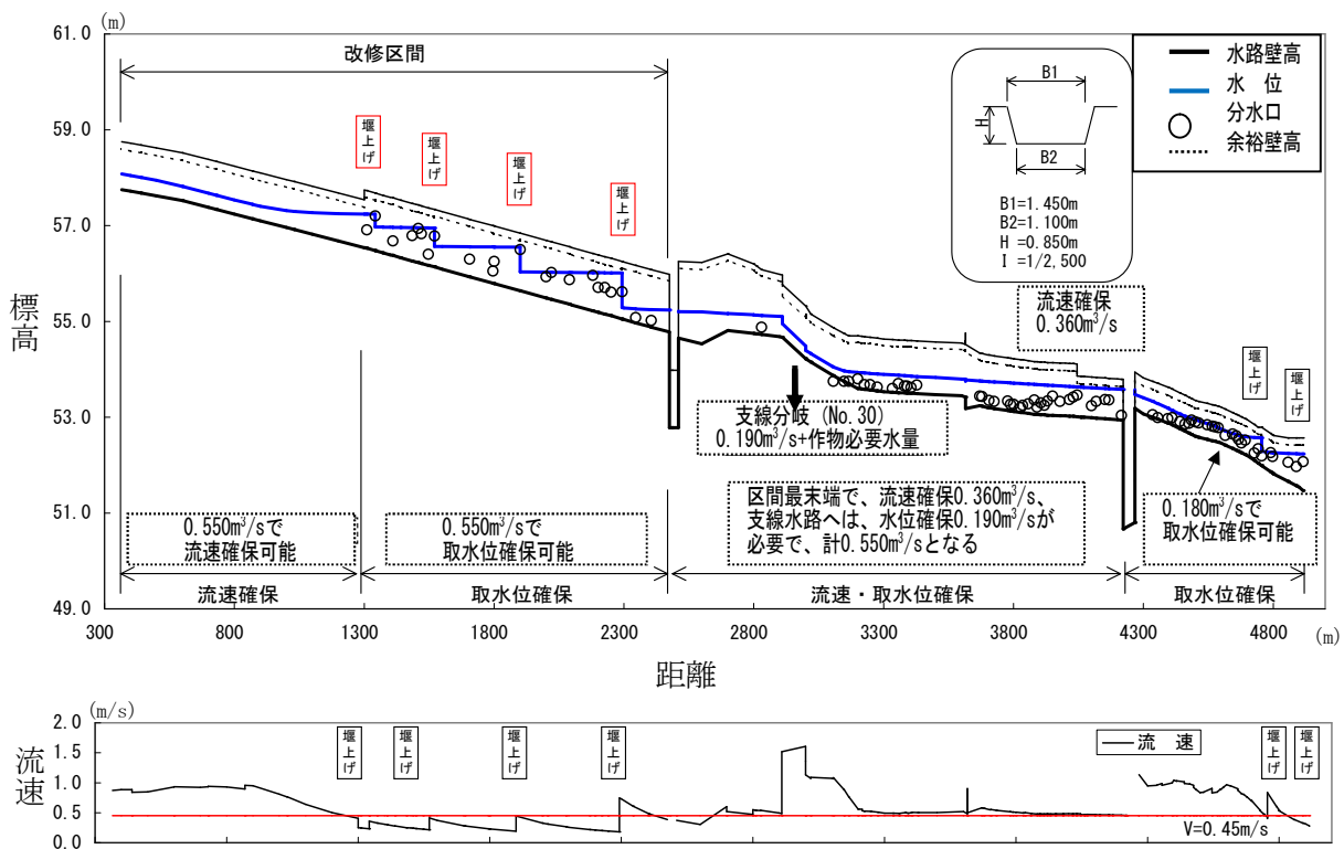
図-9.3 計画ケースでの検討結果（水位確保流量 0.550 \text{ m}^3/\text{s} ）
