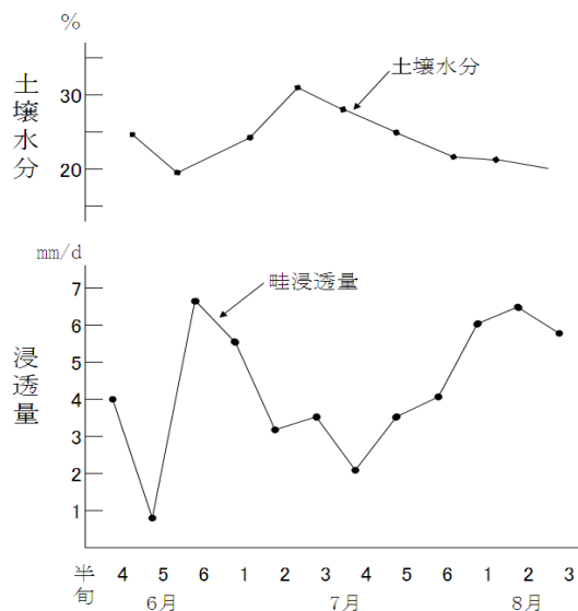
図-6.15 畦畔浸透量と土壤水分の関係
