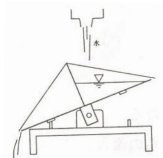
図-6.4 転倒枡の原理
