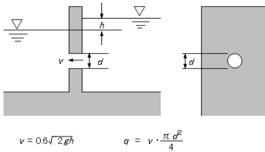
図-6.5 オリフィスによる流量測定の実験装置と原理図
