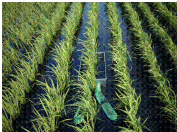
写真-6.6 N型減水深測定器設置例
