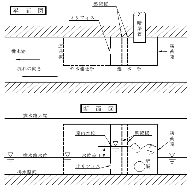
図-6.6 オリフィスによる暗渠排水量の測定装置の平面図と断面図
