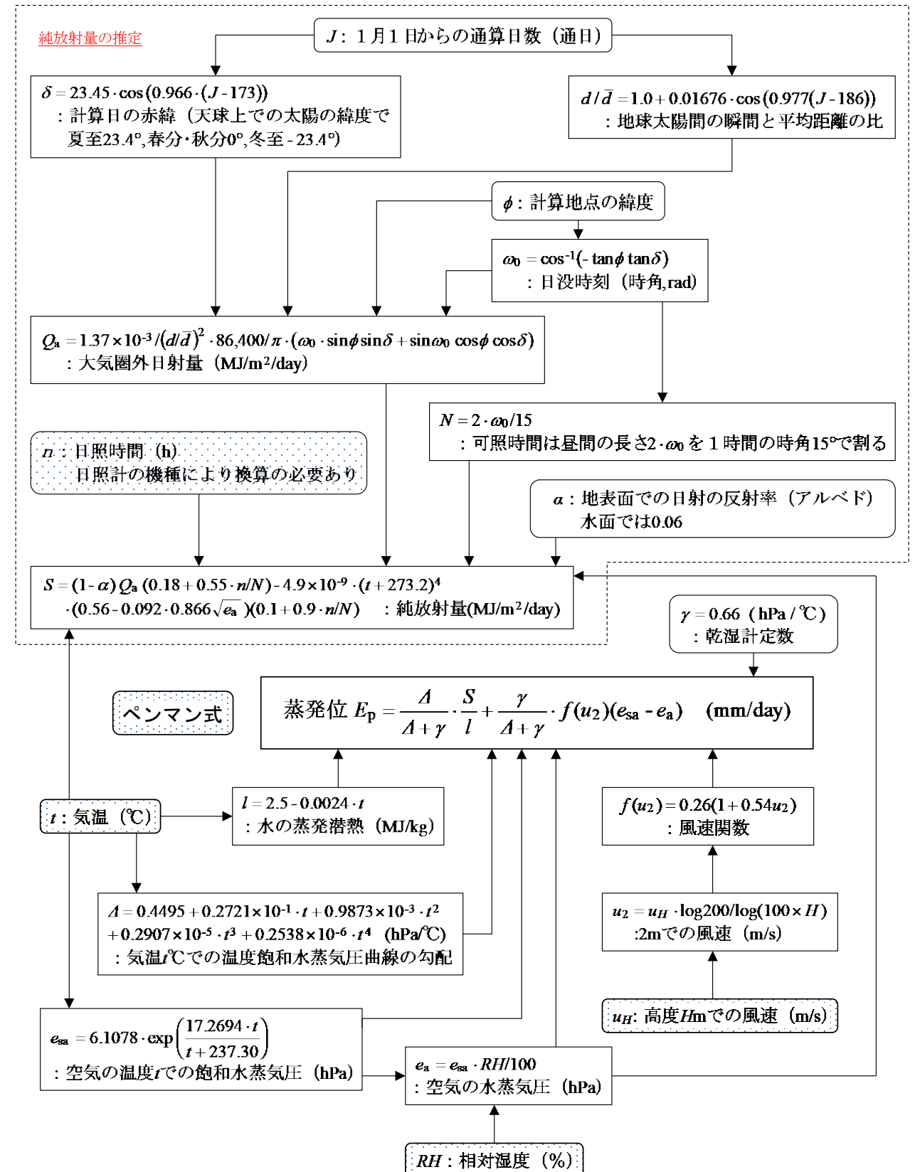
図-8.5 ペンマン式の計算手順
