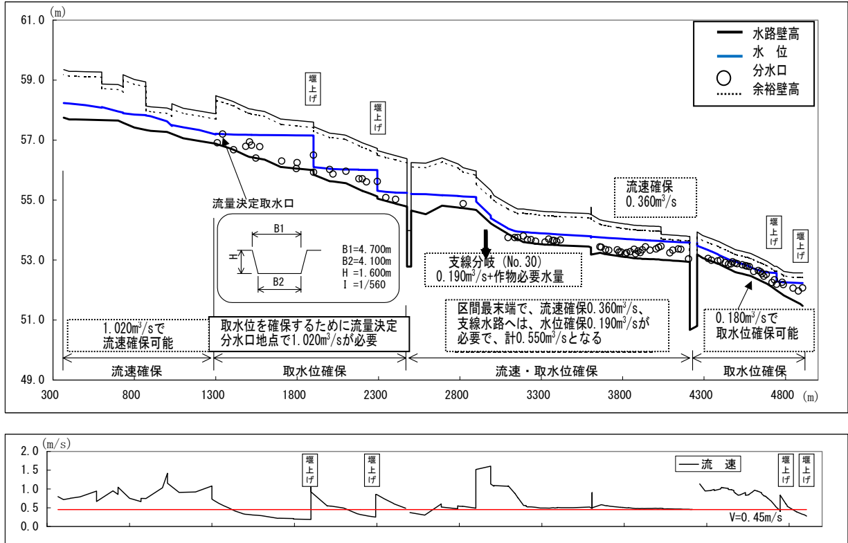
図-9.2 現況ケースでの検討結果 (水位確保流量 1.020m 3 /s)
