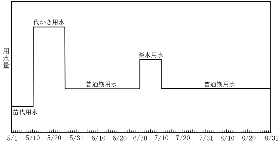
図-7.4 移植栽培での水利用パターン（北海道の事例）
