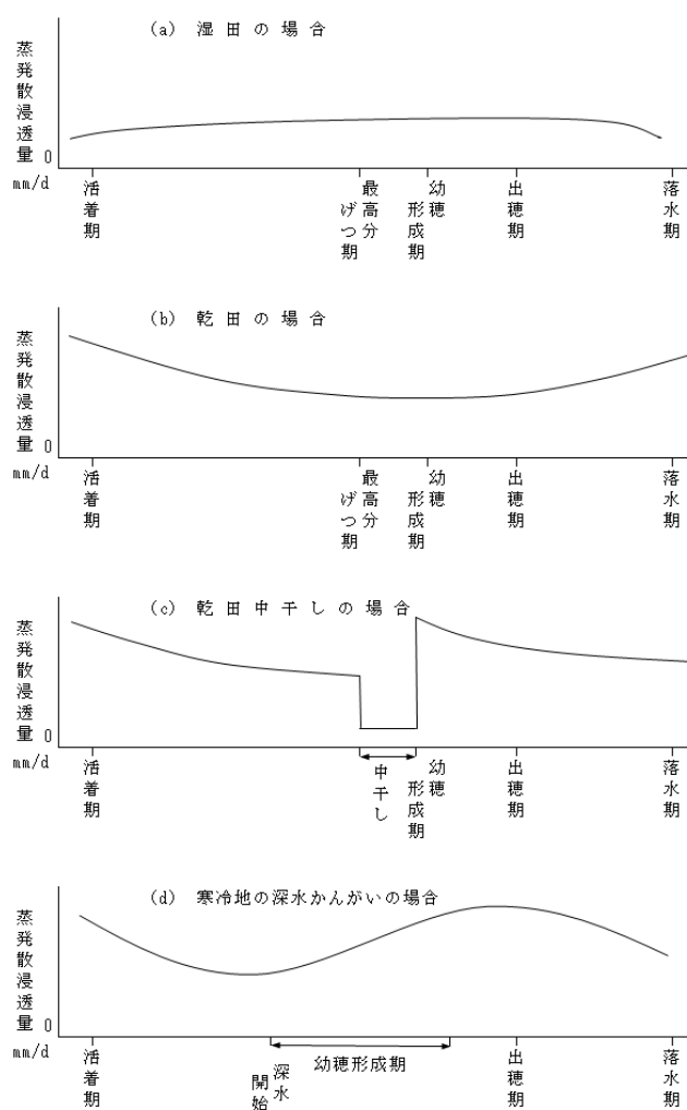
図-7.1 蒸発散浸透量の標準的期別変化の模式図
