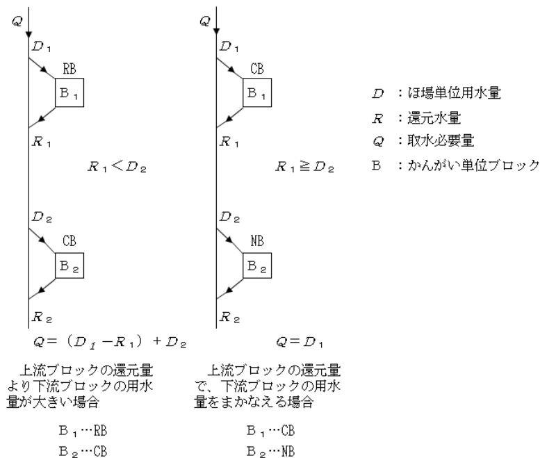
図-11.1 CB法によるブロック組合せの基本形
