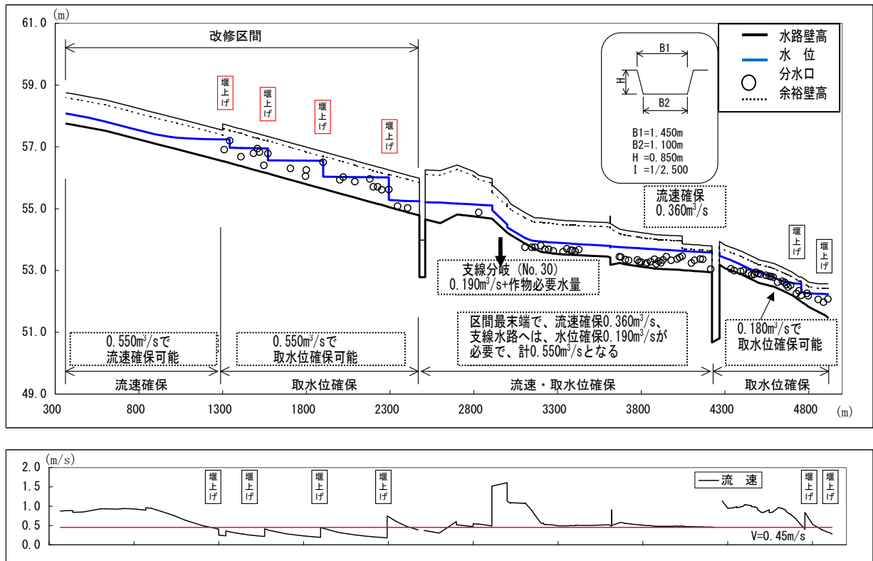
図-9.3 計画ケースでの検討結果 (水位確保流量 0.550m 3 /s)
