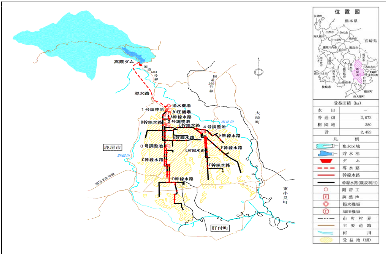
笠野原地区 概要図
