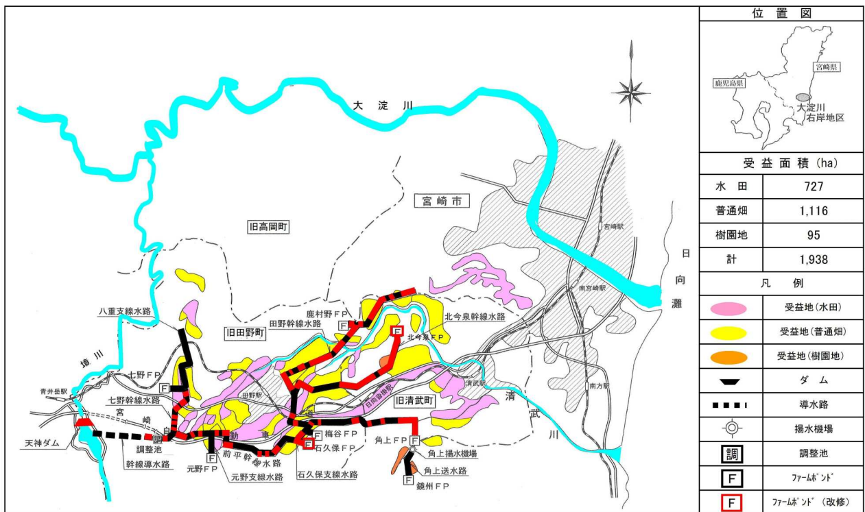
大淀川右岸地区 概要図
