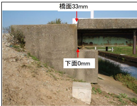
橋台の傾き (桁と橋台の隙間の測定)
