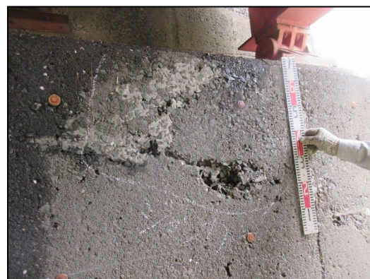
骨材の偏在による空隙
