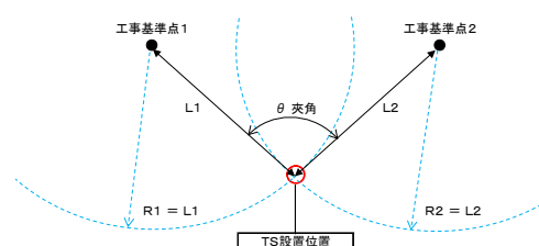
図 20 後方交会法
