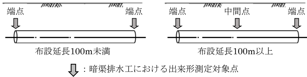
図6 出来形計測箇所（暗渠排水工）
