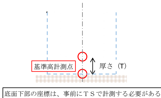
図 12 厚さの計測
