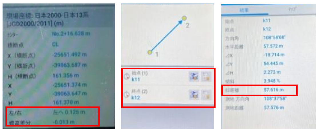
図1 出来形確認画面例
