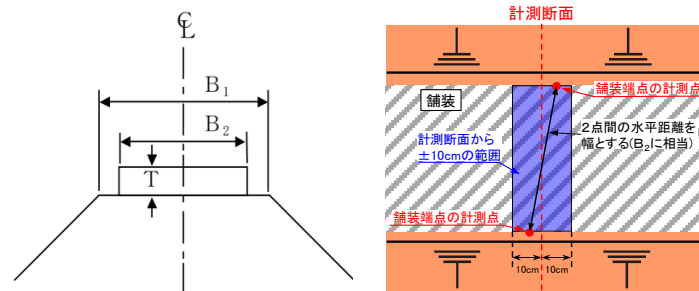
図2-1 出来形測定箇所標準図（左：横断面、右：平面図）
