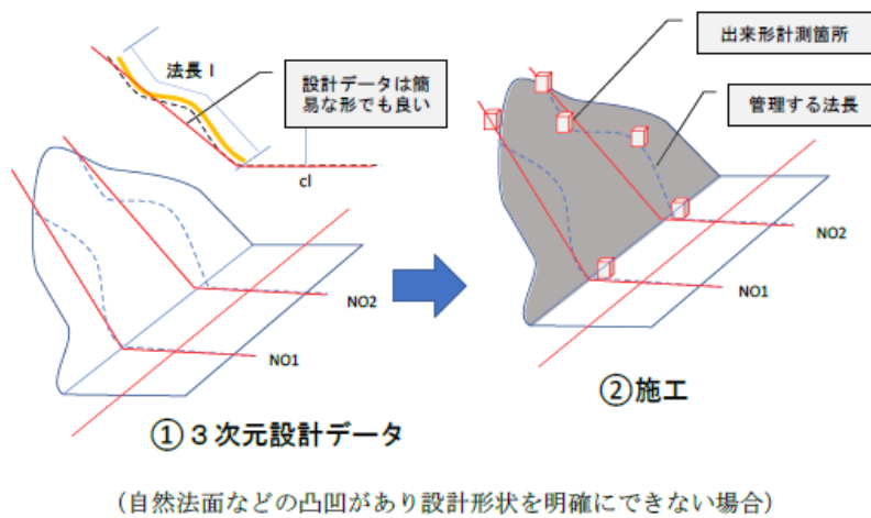
図8 出来形計測箇所（法面保護工）
