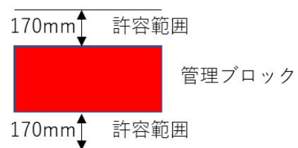
図 5 - 6 水平離隔の良否基準イメージ
