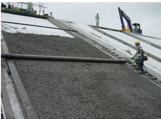
③ストライカーチューブによる敷き均し
