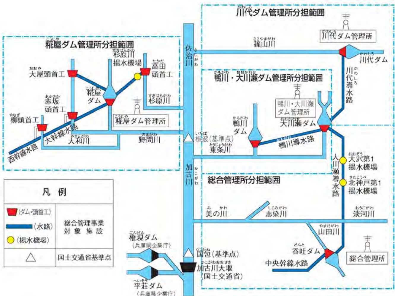
<加古川水系地区の系統模式図>
