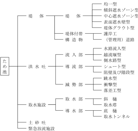
図 1-1 ため池の施設構成
