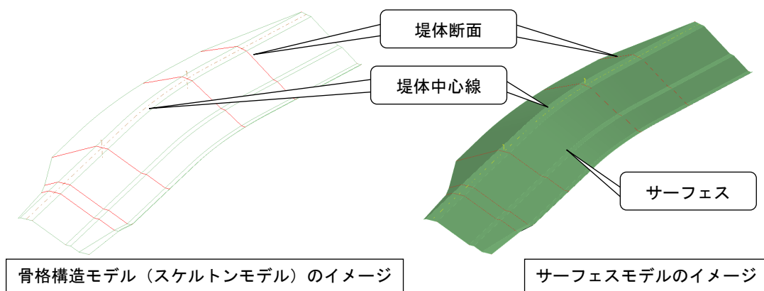
図 3-6 骨格構造モデル（スケルトンモデル）とサーフェスモデルの例（堤体）
