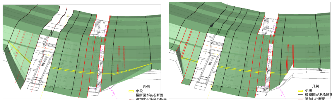
図 3-4 断面変化箇所の断面追加例
