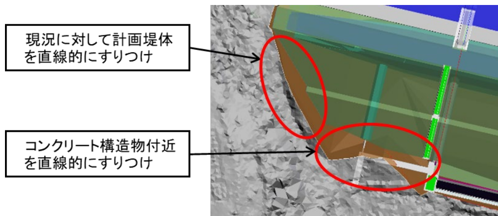
図 3-3 堤体袖部すり付け例
