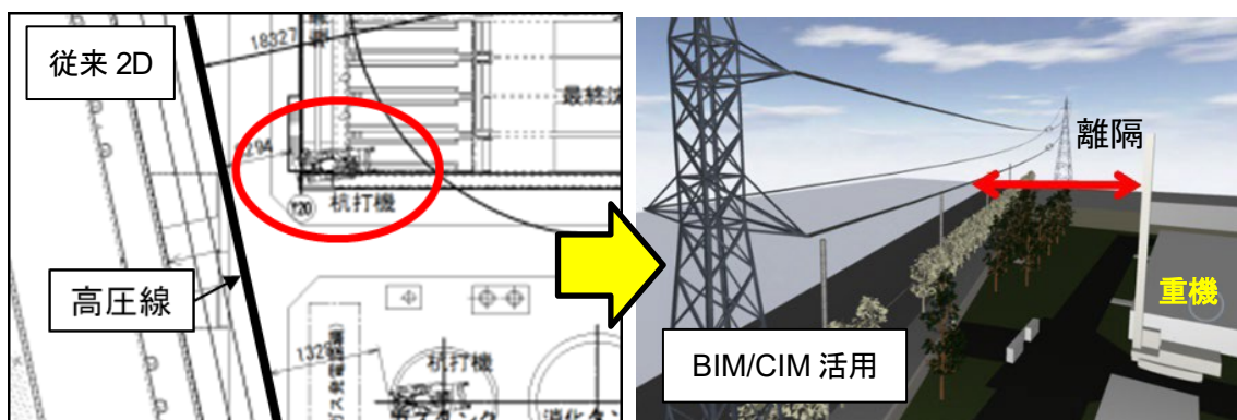
図 3-2 電力会社との近接協議に活用した例
