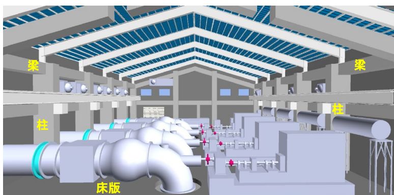
図 3-5 各部材によるモデル作成例
