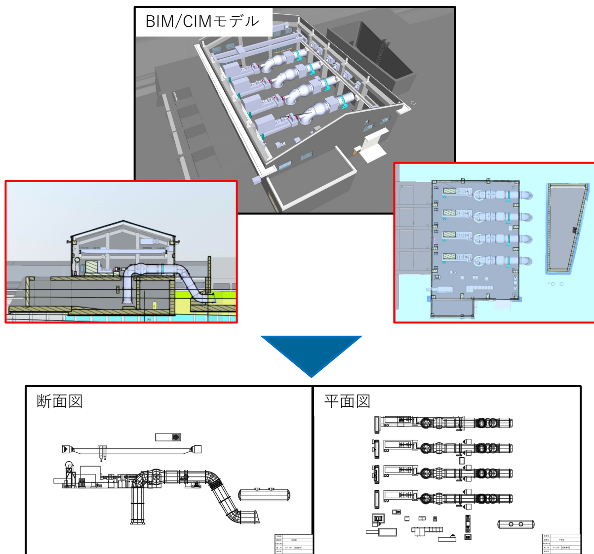
図 3-3 BIM/CIM モデルから作成した 2 次元図面の例
