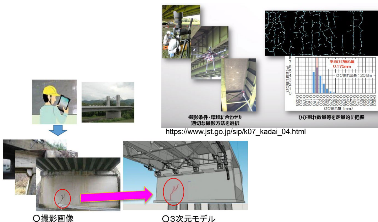
図 3-4 点検調査結果を 3 次元モデルへ適用した例
