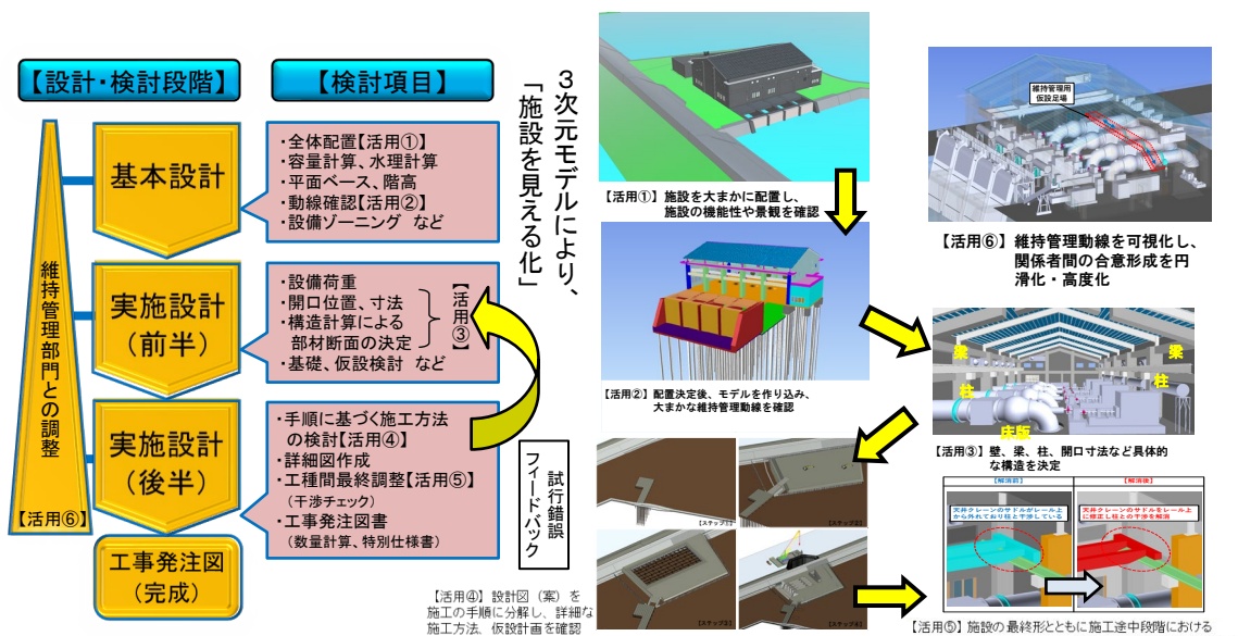
図 3-1 設計業務の作業フロー
