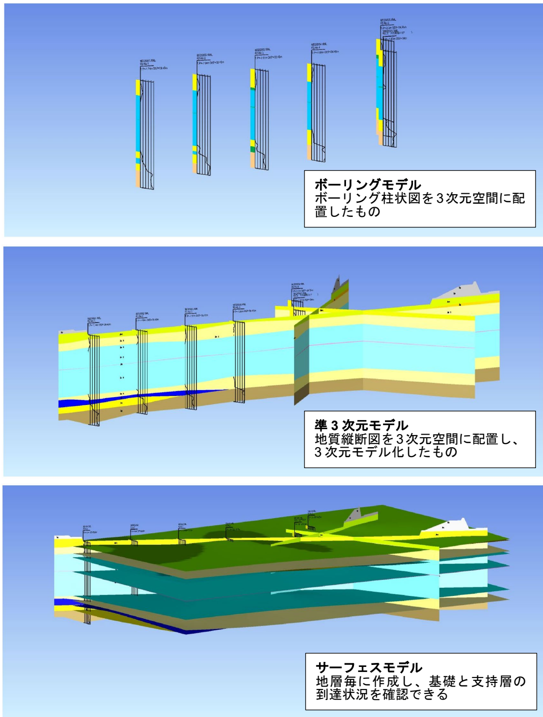
図 2-1 地質・土質モデルの作成例
