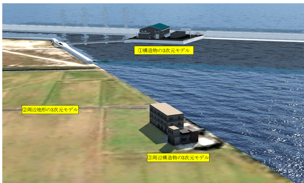
図 3-6 ポンプ場における BIM/CIM モデルの構成例
