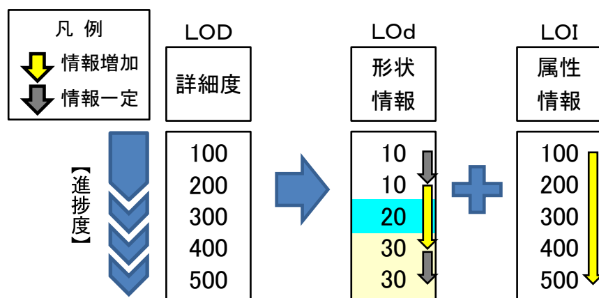
図 1-10 機械設備モデル（機器類）の詳細度設定の例
