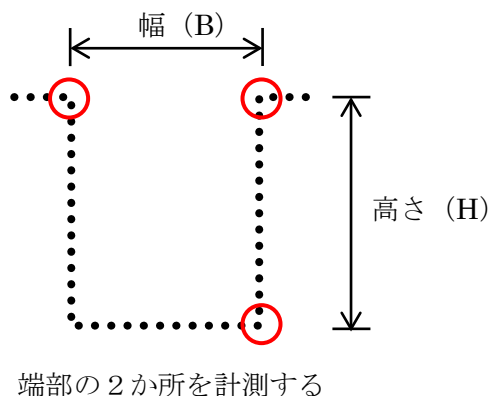
図4-6 幅、高さの計測
