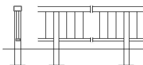
高欄構造形式図
