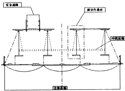
【床版足場】：主体足場 * ＋朝顔＋床版足場補強
