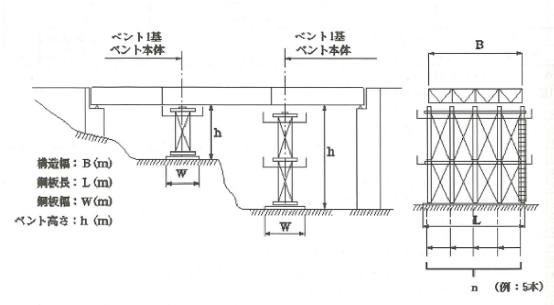
ベント設備 (参考図)
