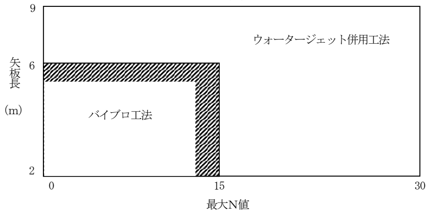
図 3. 1 工法選定図
