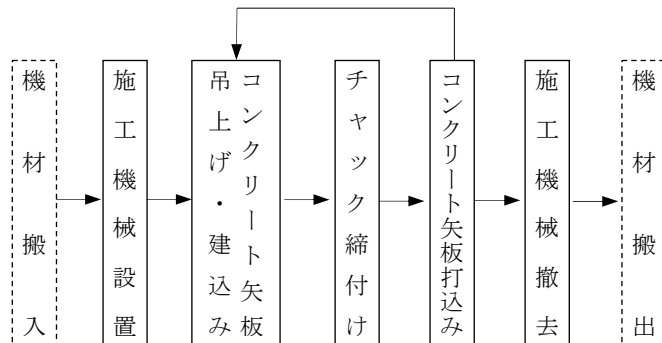
図2-1 バイブロ工法
