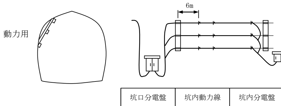
図１ 動力線布設図
