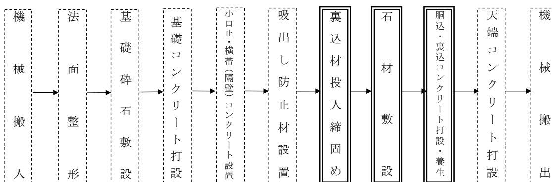
図 2-1 施工フロー
